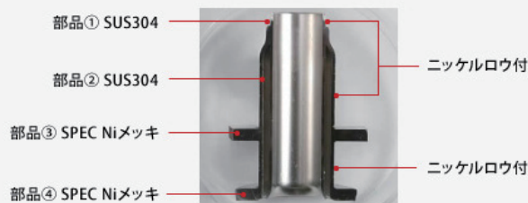
4部品を組付、ニッケルろう材で一体化ろう付加工
