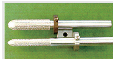
4部品を組付、ニッケルろう材で一体化ろう付加工
